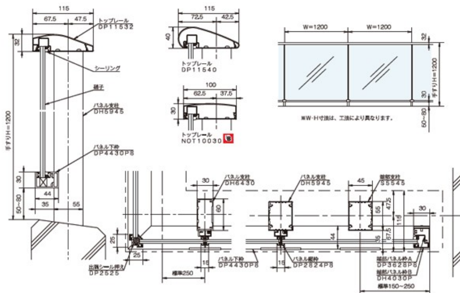
【断面図】SL-FRI-NOT10030-45(30)
