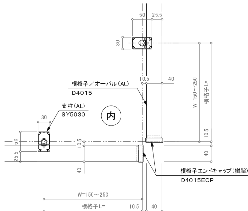
出隅コーナー(2)平面詳細図 S=1/6
