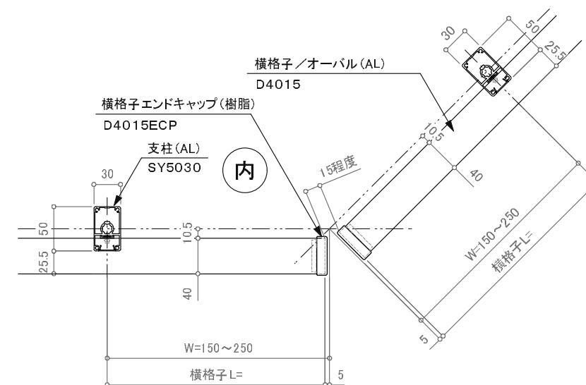
出隅135度コーナー平面詳細図 S=1/6
