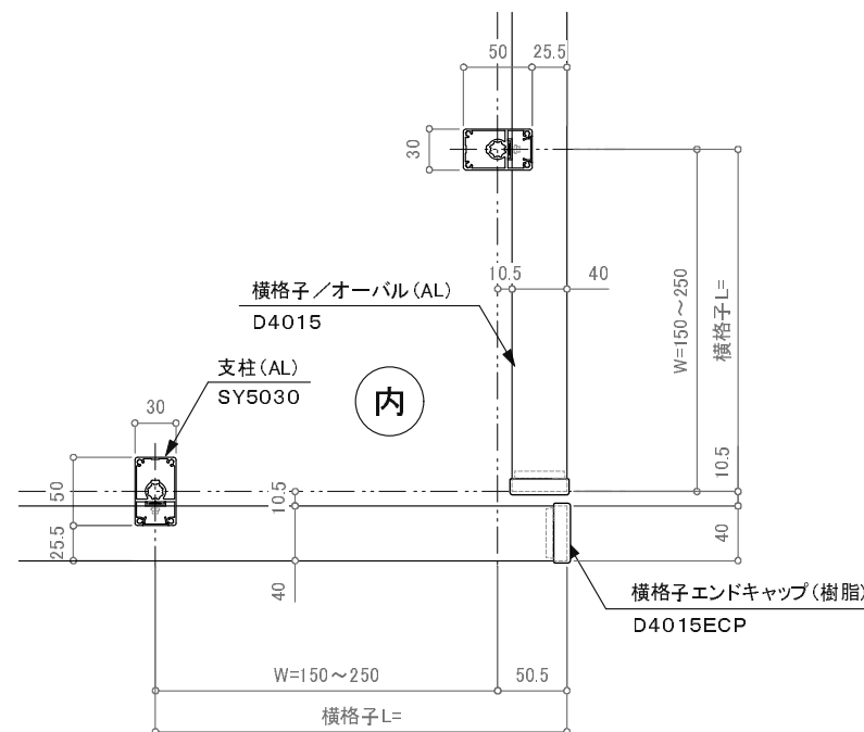
出隅コーナー(1)平面詳細図 S=1/6
