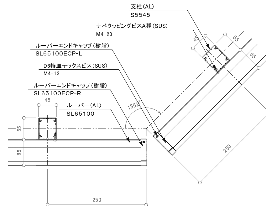
出隅135度コーナー平面詳細図 S=1/6
