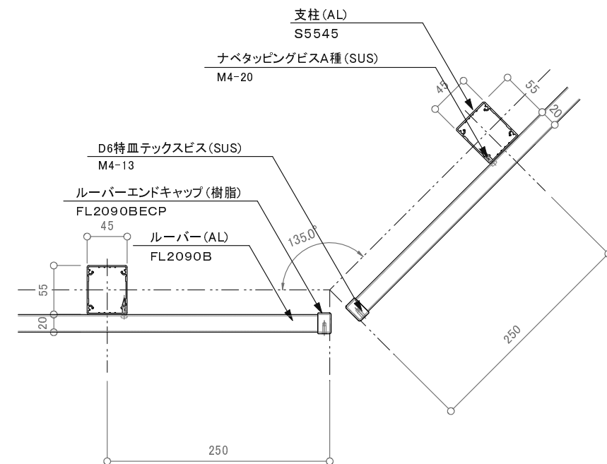
出隅135度コーナー平面詳細図 S=1/6
