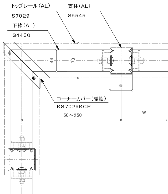
ドレンコーナー納まり S7029
