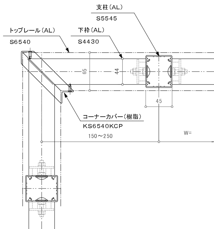
ドレンコーナー納まり S6540
