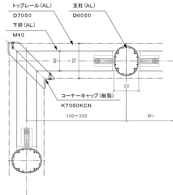
ドレンコーナー納まり D7050
