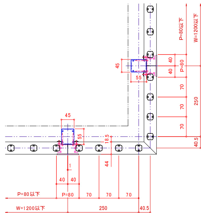
ドレンコーナー (250×250) 格子ピッチ80の場合
