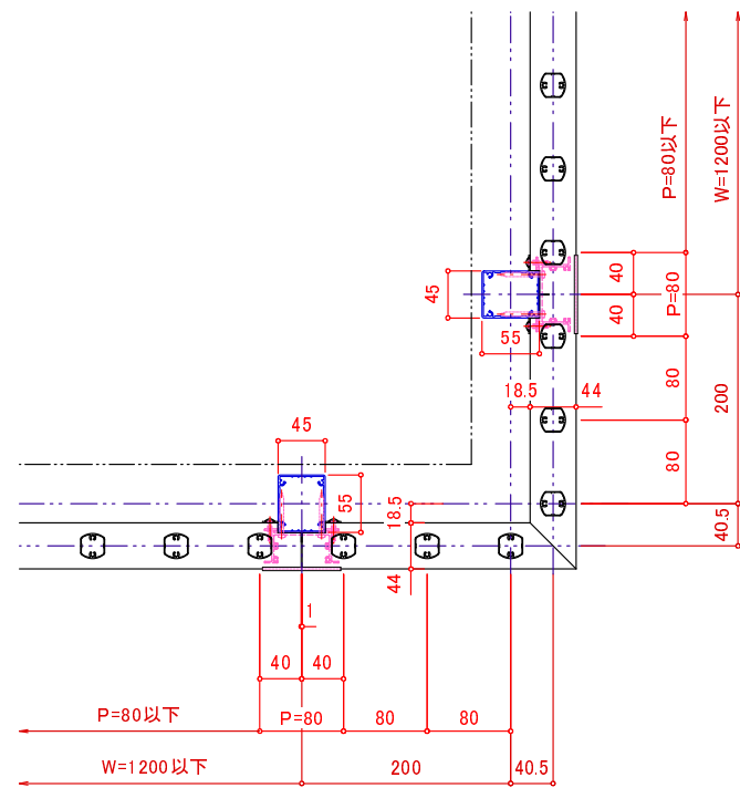
ドレンコーナー (200×200) 格子ピッチ80の場合
