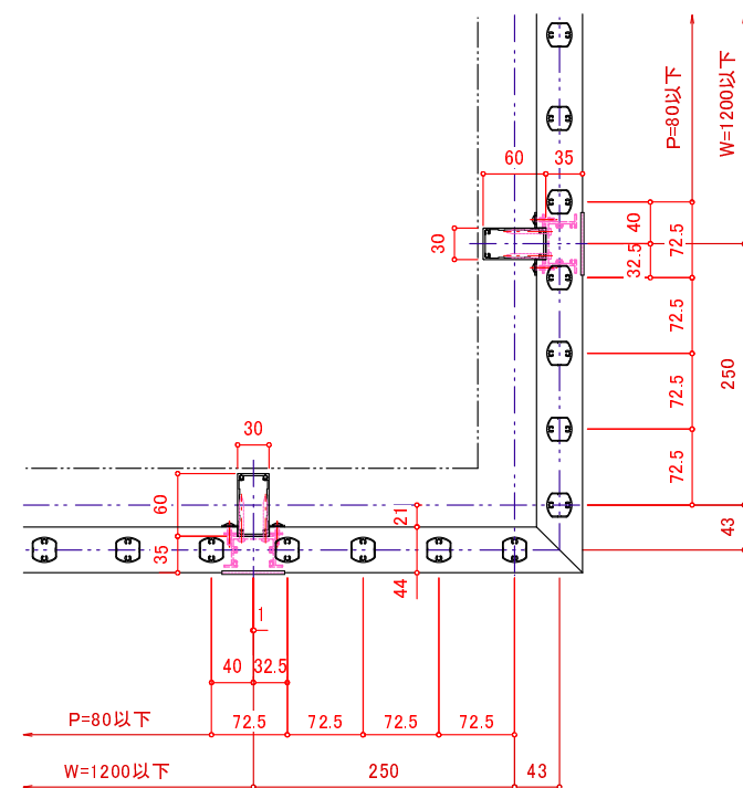
ドレンコーナー (250×250) 格子ピッチ80の場合
