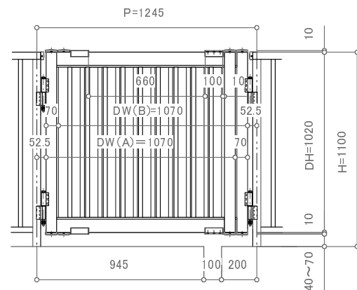
ストローク300の場合の参考立面図(-300)
