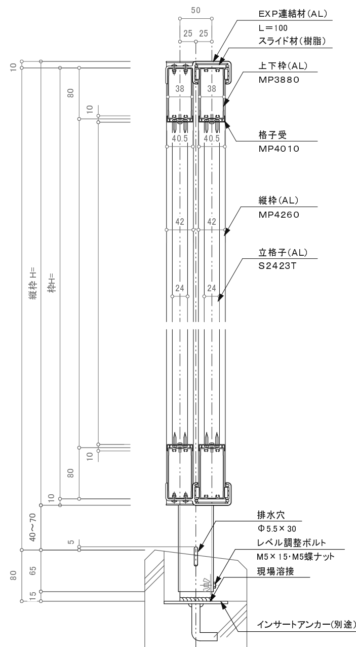
ストローク300の場合の参考立面図(-300)
