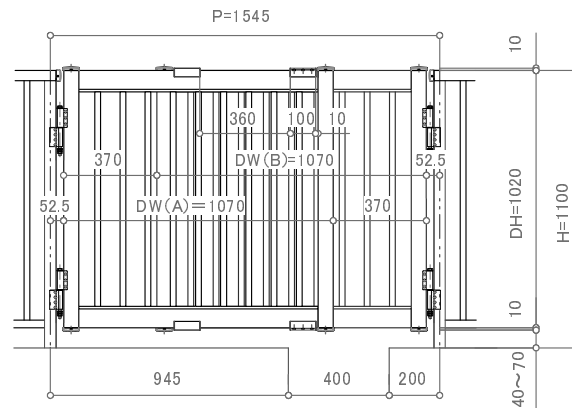
ストローク300の場合の参考立面図(±0)
