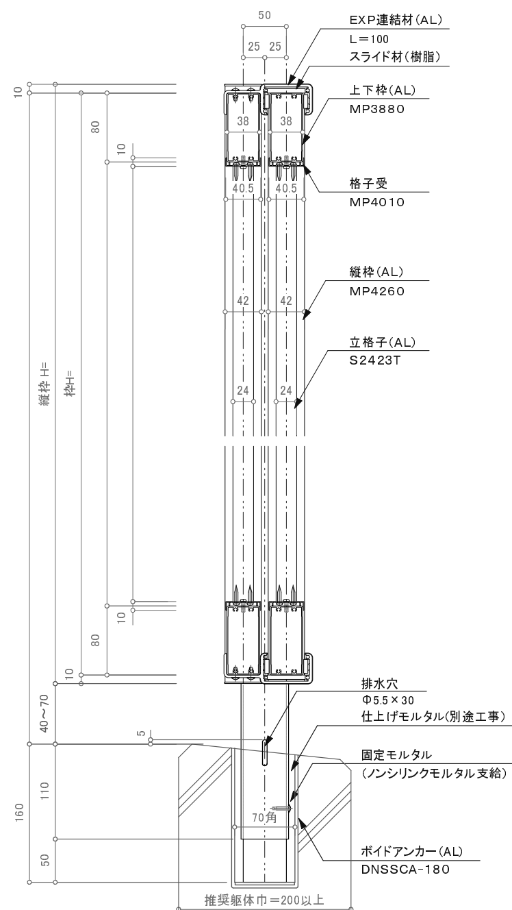
ストローク300の場合の参考立面図(-300)
