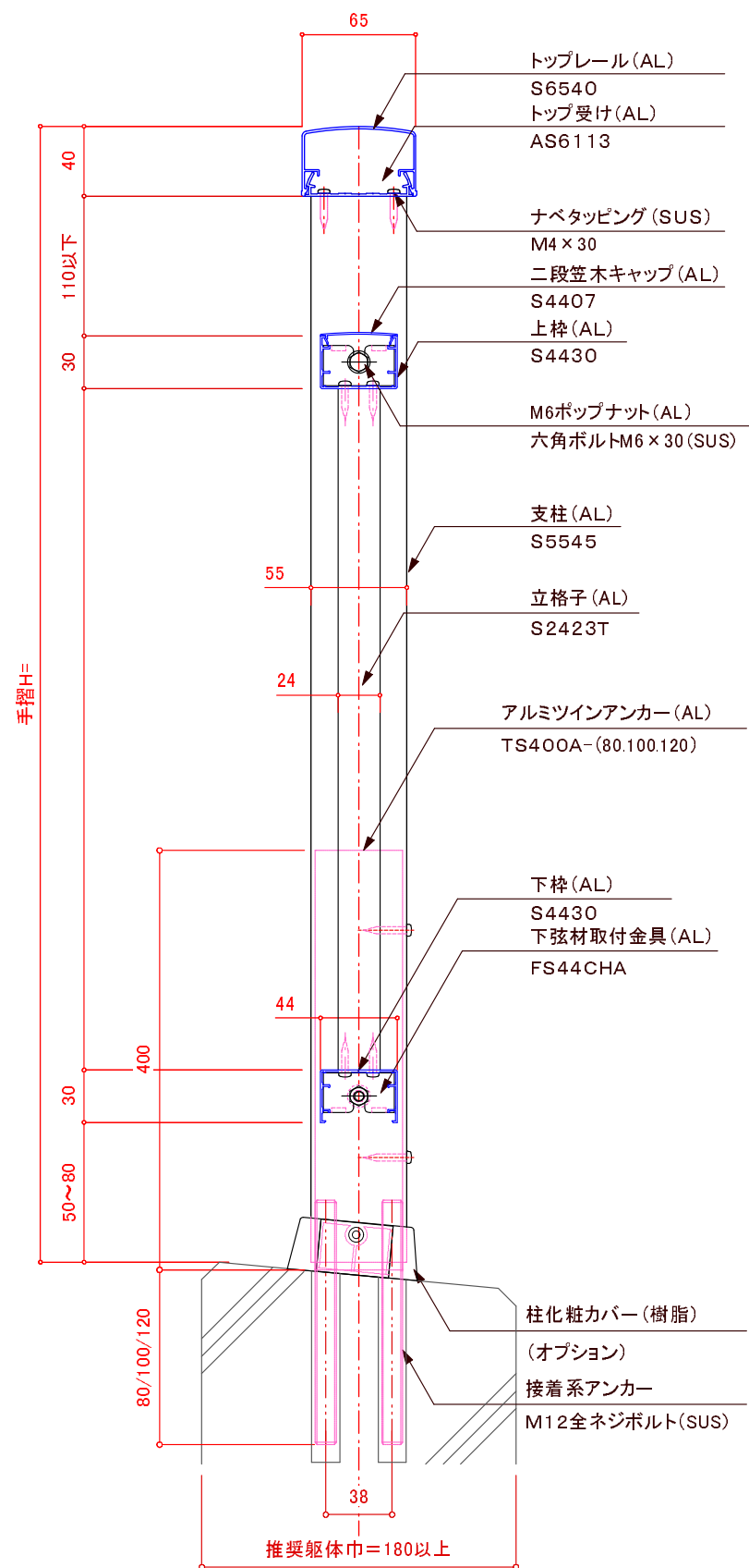
断面図
