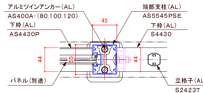
パネルと立格子の連結部詳細図
