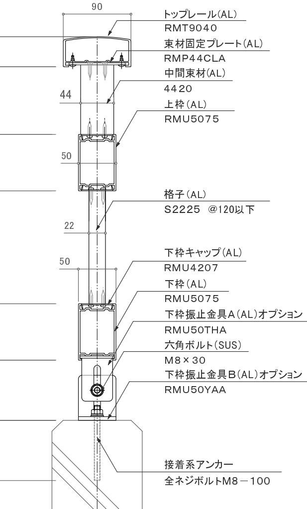
中間支持部 断面図 S=1/5
