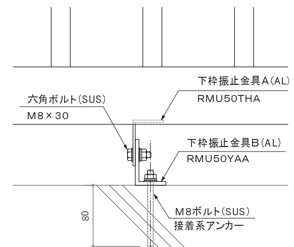
下枠振止金具部(オプション) 詳細図 S=1/5
