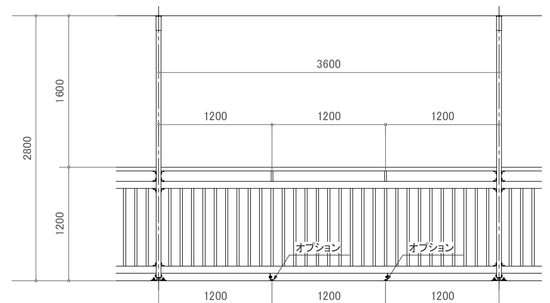
姿図 S=1/40
