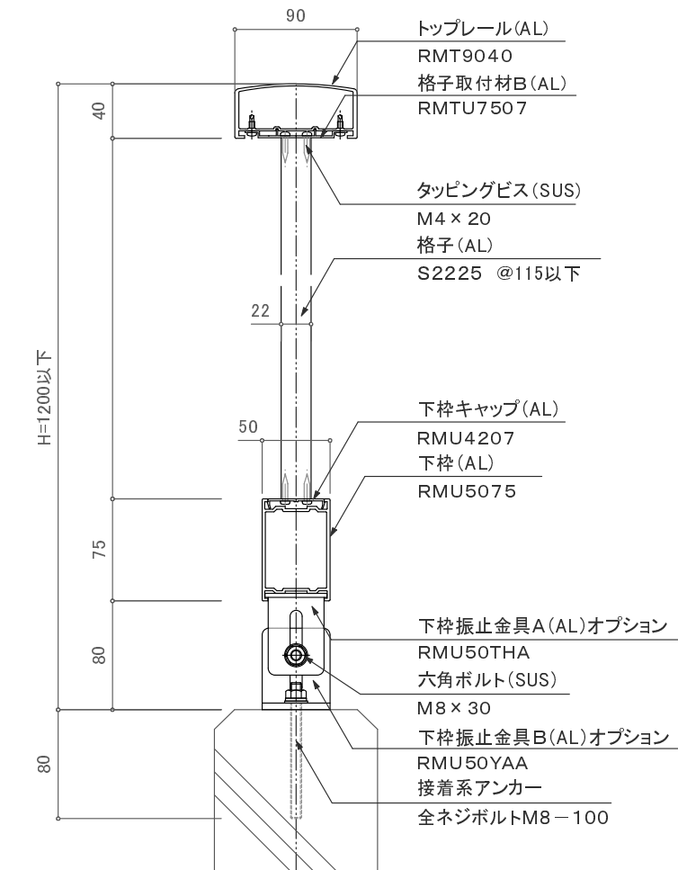
中間支持部 断面図 S=1/5
