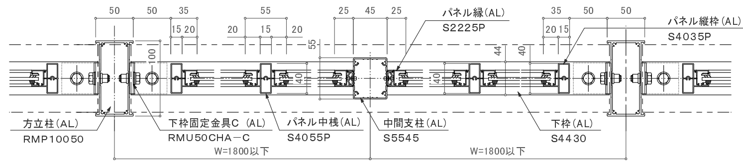
平面図 S=1/5
