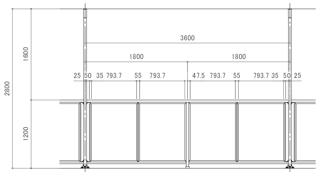
姿図 S=1/40
