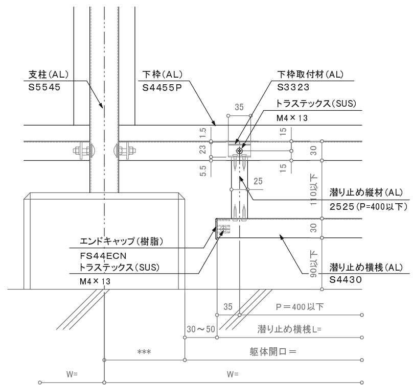
立面詳細図
