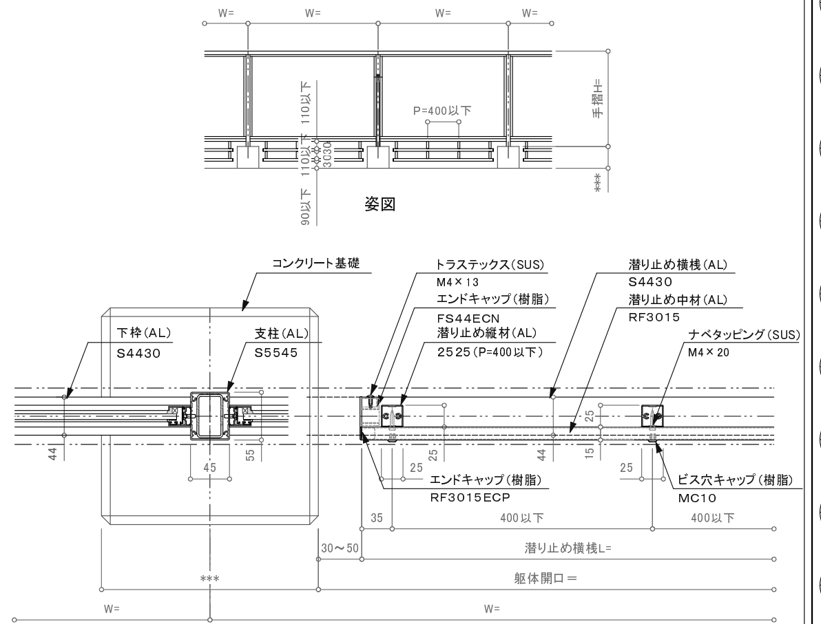
平面詳細図
