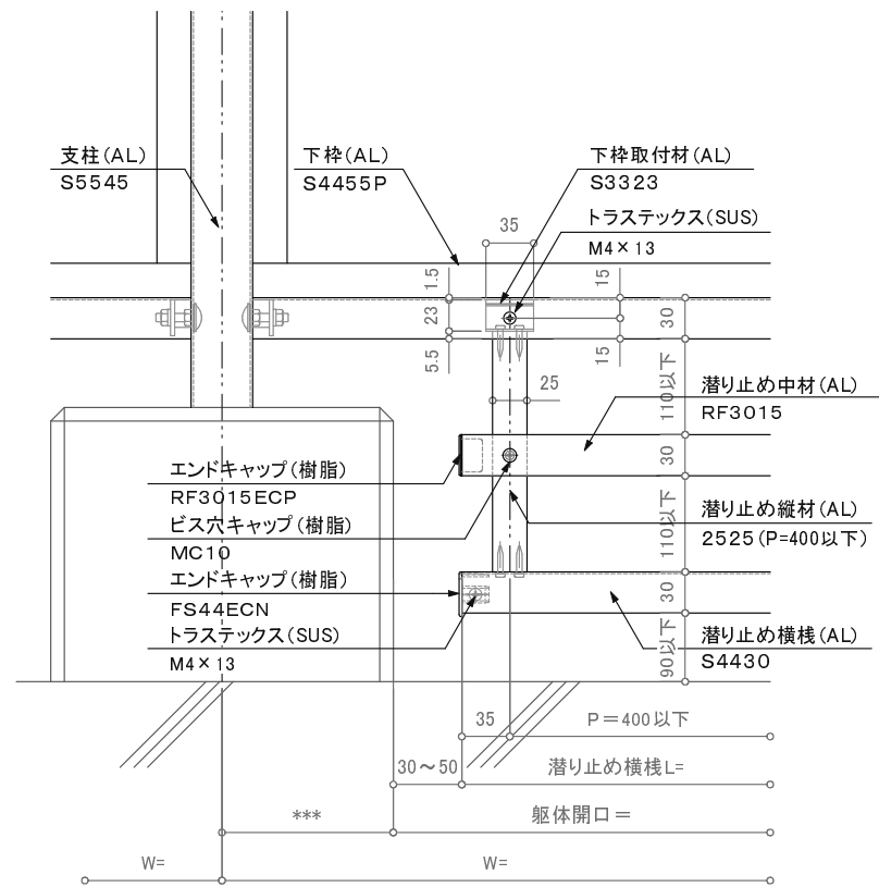
立面詳細図
