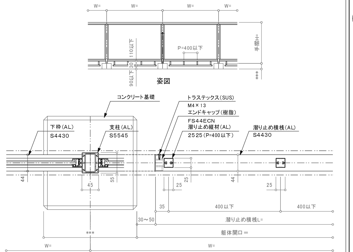
平面詳細図
