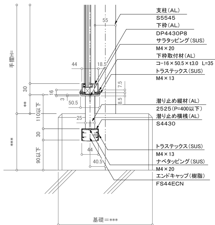
訂正 下枠DP4430P8の場合／潜り止めS4430一段タイプ 断面図
