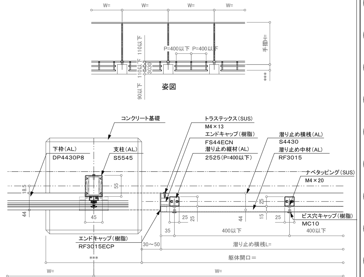
平面詳細図
