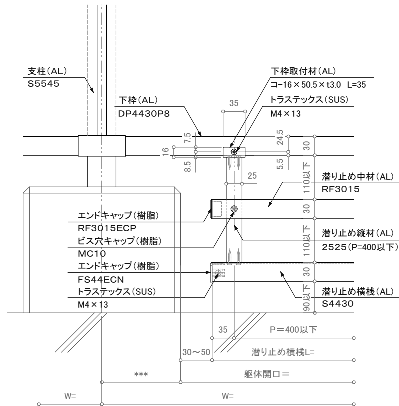
立面詳細図
