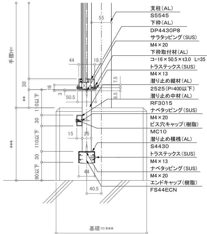
下枠DP4430P8の場合／潜り止めS4430二段タイプ 断面図
