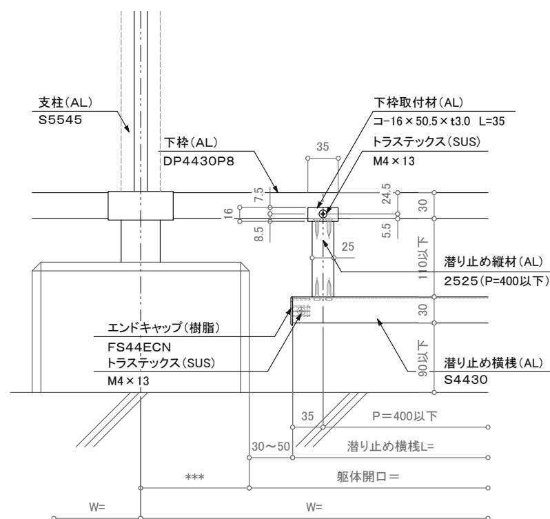
立面詳細図
