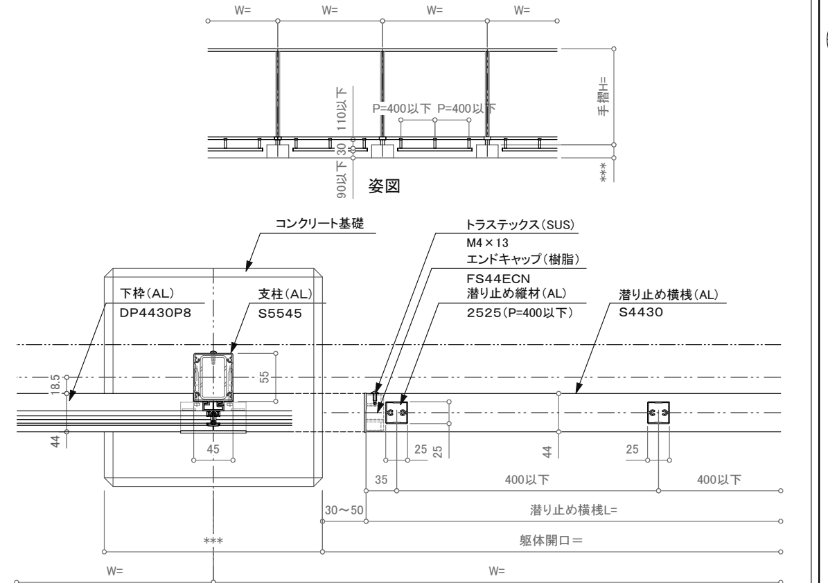
平面詳細図
