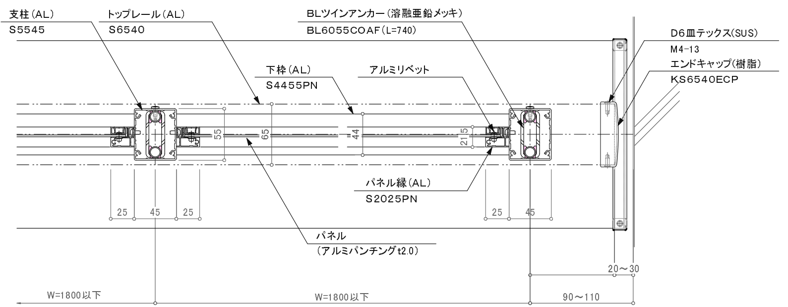
バルコニー用150型／KBK-2BW (一 体 型)
