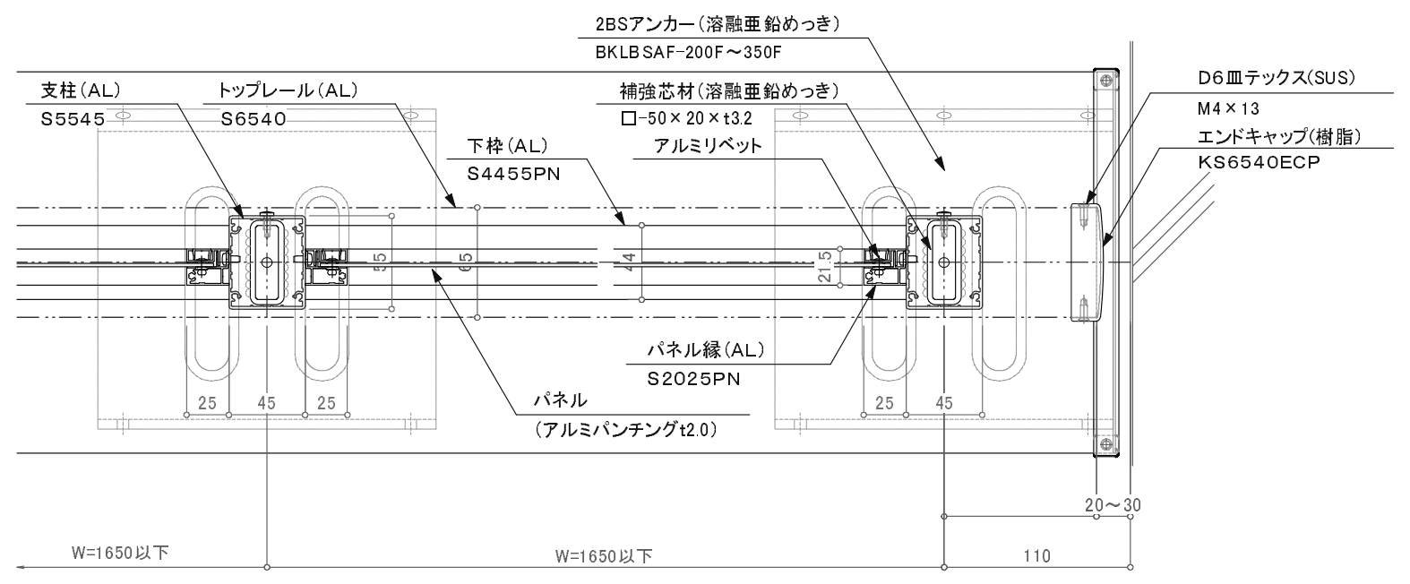
バルコニー用150型／KBK-2BS
