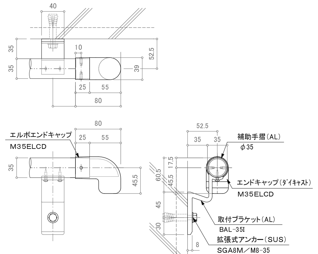
エルボエンドキャップ仕様(下向き) 詳細図
