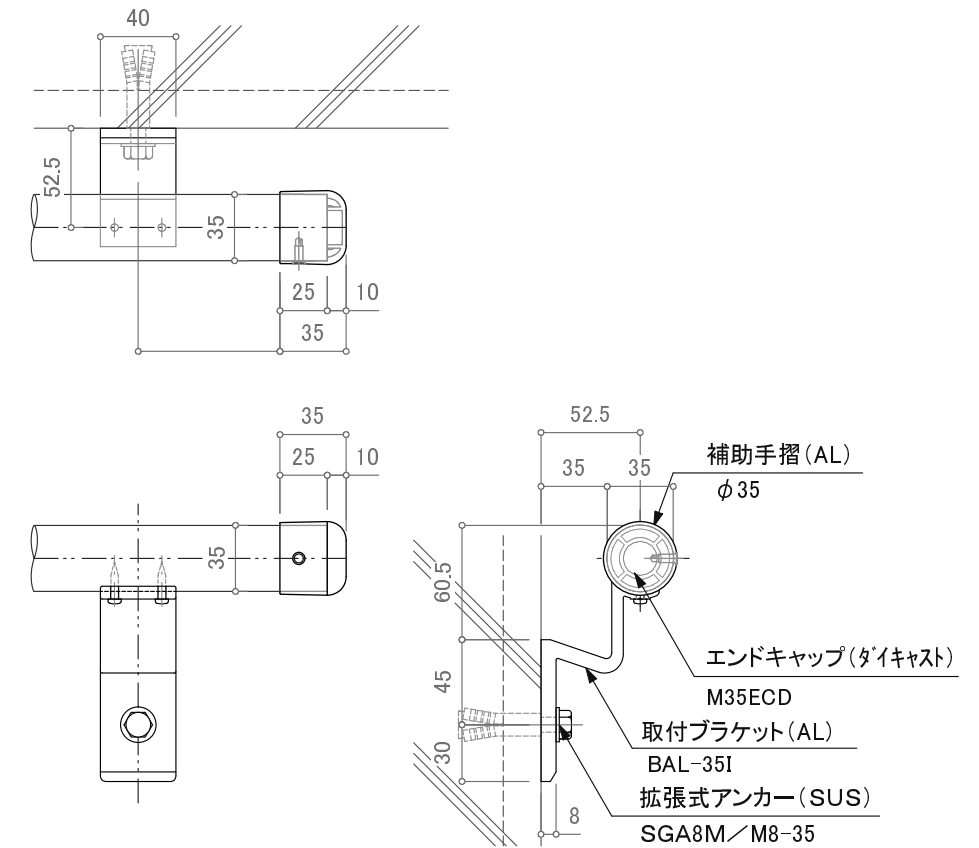
エンドキャップ仕様 詳細図
