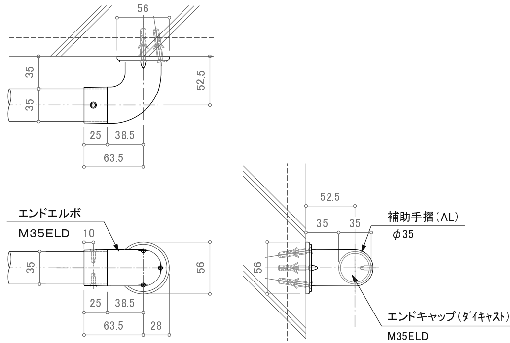
エルボエンドキャップ壁支持仕様 詳細図
