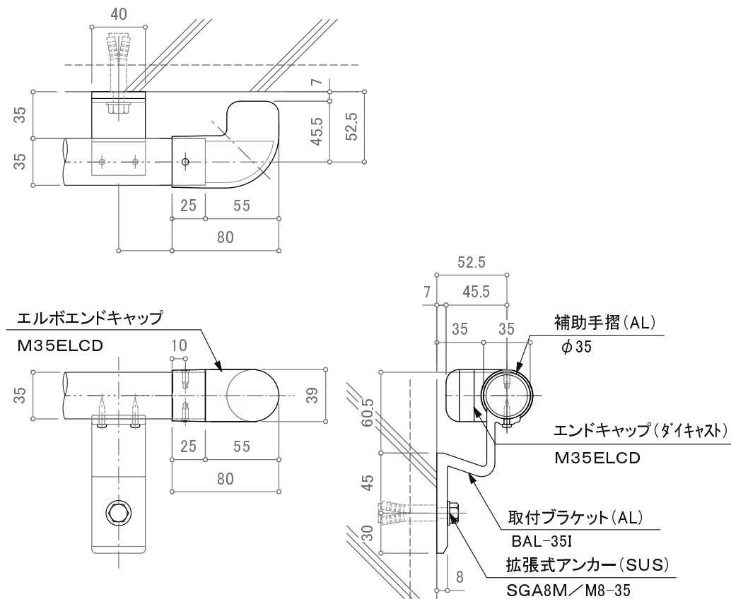
エルボエンドキャップ仕様(横向き) 詳細図
